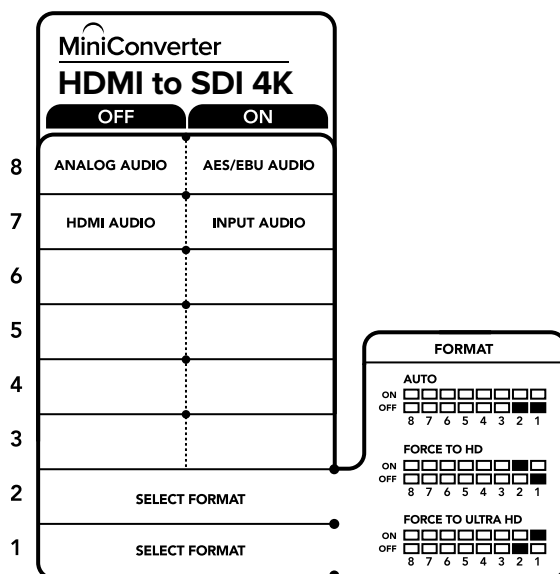
转换器背面印有开关示意图, 图中详细介绍了更改转换设置所需的全部信息。
