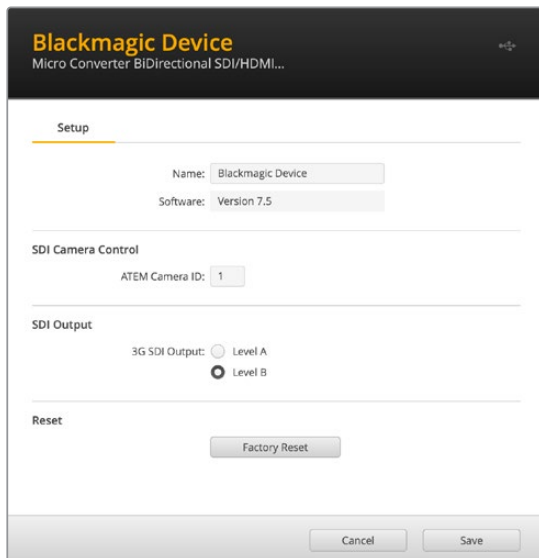
Opciones de configuración para el modelo Micro Converter BiDirectional SDI/HDMI 3G
