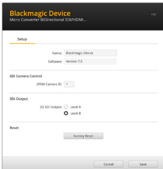
Настройки на вкладке Setup для устройства Micro Converter BiDirectional SDI/HDMI 3G
