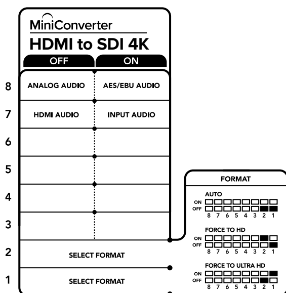
Lo schema alla base del dispositivo mostra tutte le combinazioni delle impostazioni di conversione.
