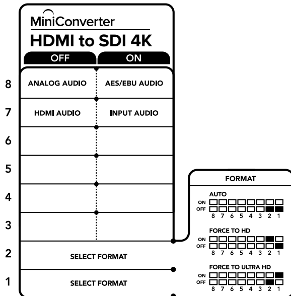
Die Switch-Legende am Boden Ihres Konverters gibt Ihnen alle erforderlichen Informationen, um die Umwandlungseinstellungen zu verändern
